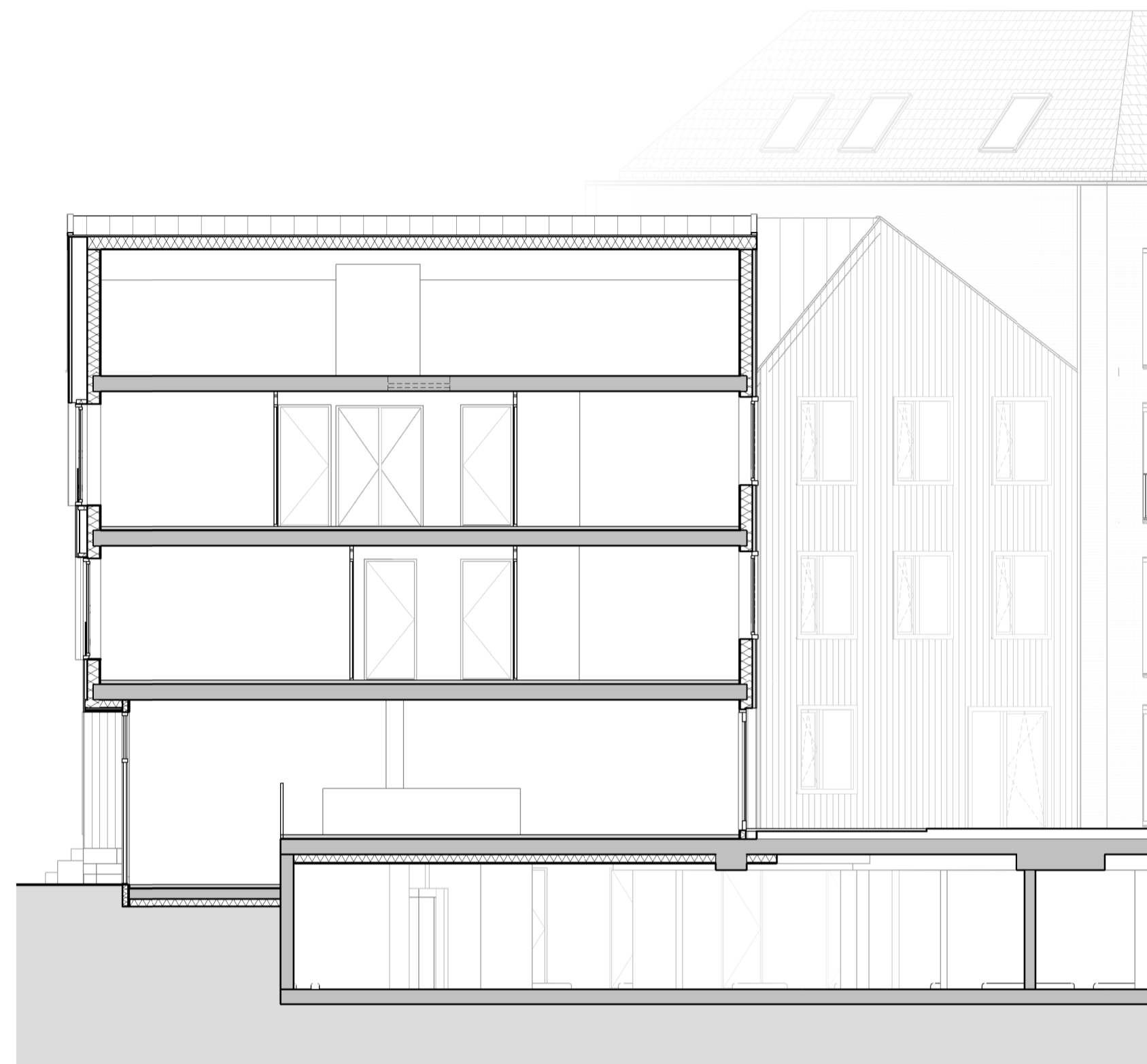
doorsnede A-A
