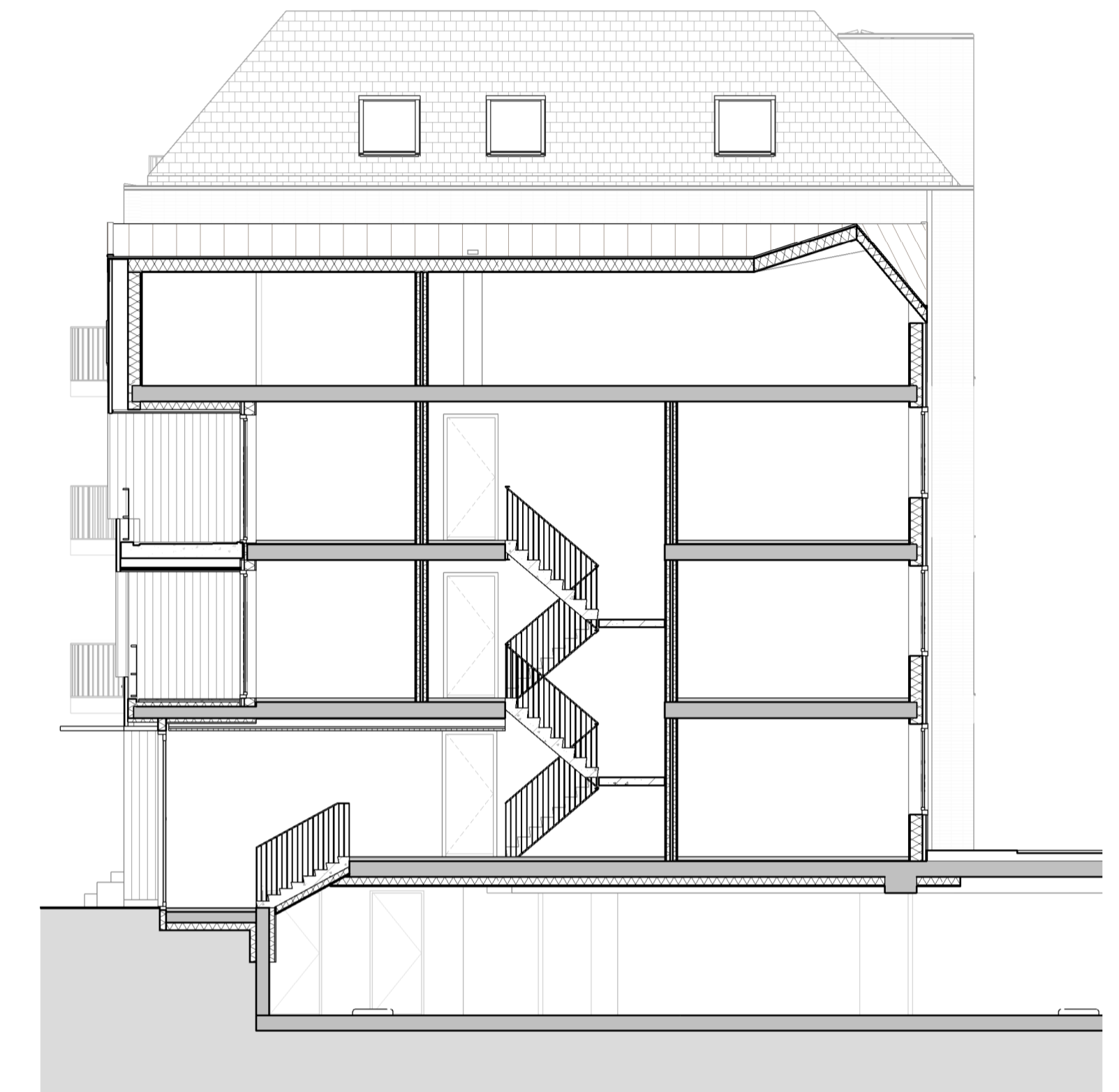
doorsnede C-C
