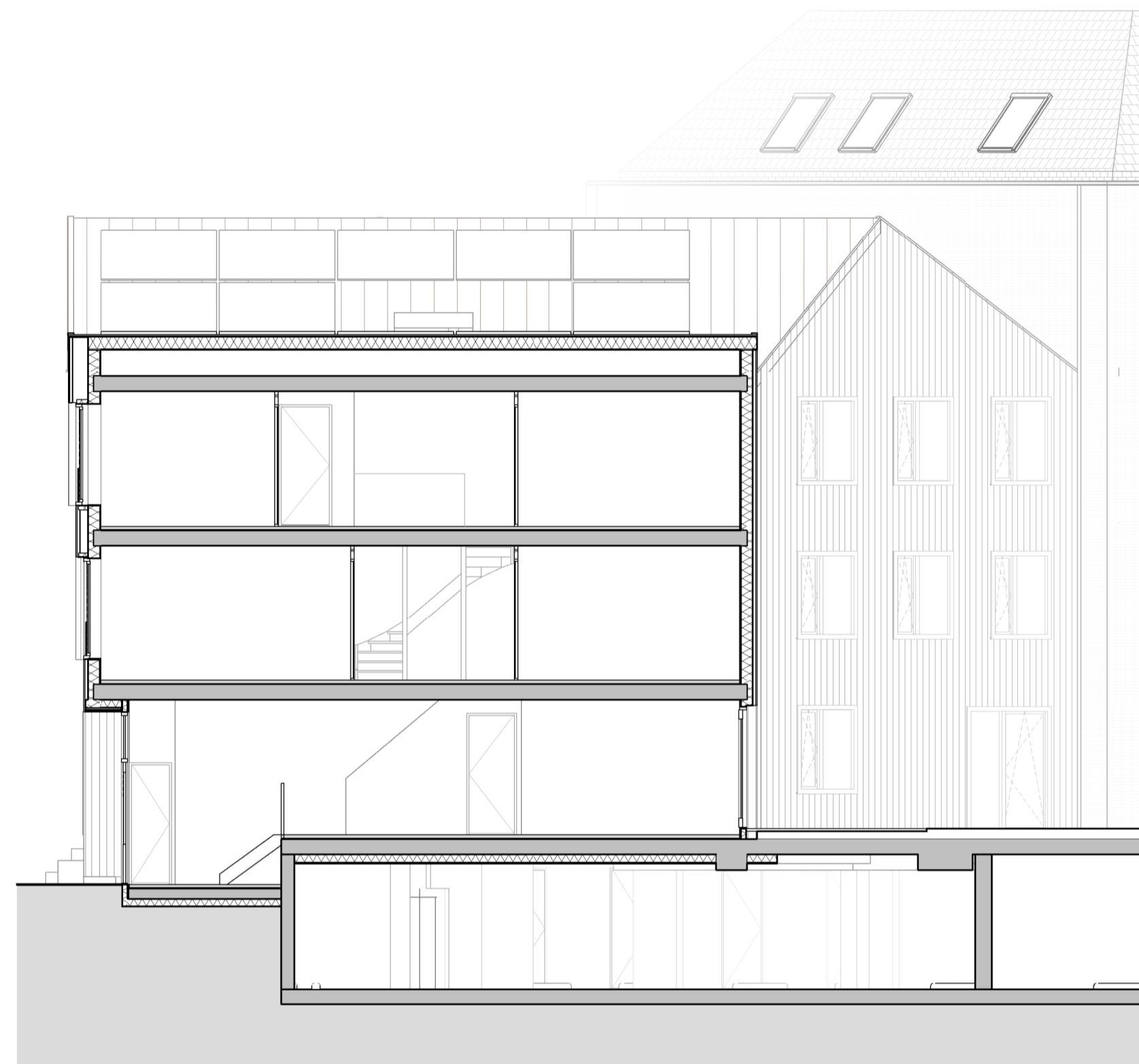
doorsnede B-B
