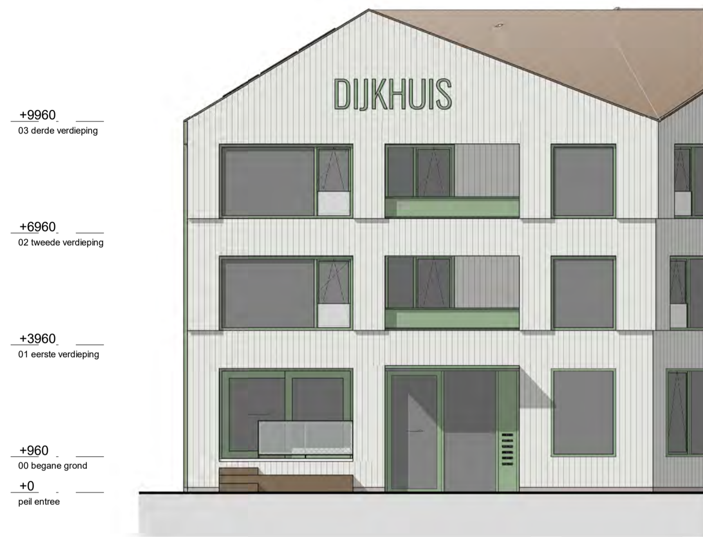
voorzijde kade
